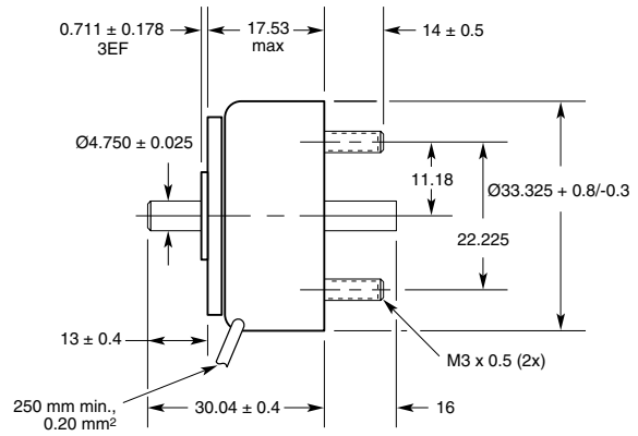
Size 3EFM/3ECM
